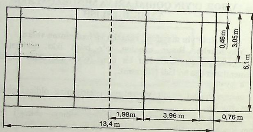
71-rasm. Kombinatsiyalangan badminton maydonchasining o'lchamlari.
